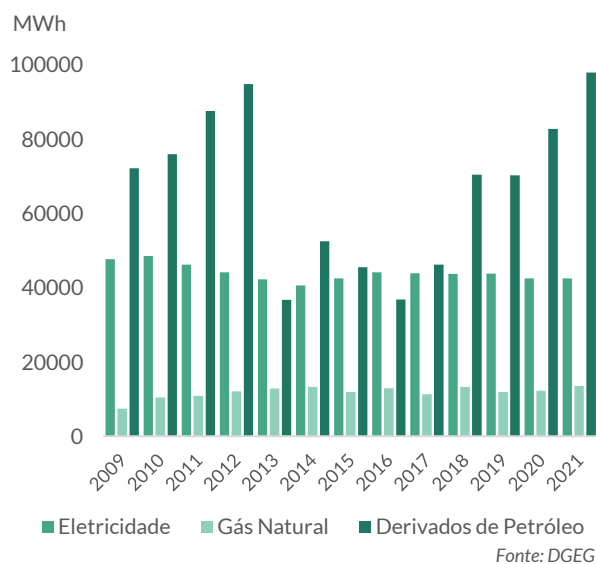
Gráfico 27 | Evolução do consumo de energia por tipo de vetor em Macedo de Cavaleiros, 2009-2021
