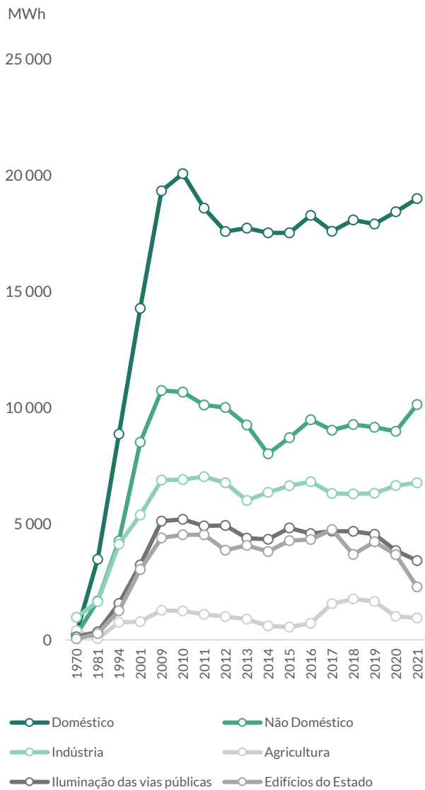
Gráfico 30 | Evolução do consumo de energia elétrica por tipo de consumo em Macedo de Cavaleiros, 1970-2021
