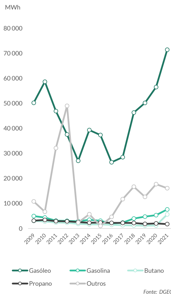
Gráfico 28 | Evolução do consumo de combustíveis derivados de petróleo, em Macedo de Cavaleiros, 2009-2021
