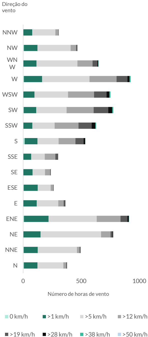
Gráfico 10 | Número de horas de vento por ano, velocidade e direção em Macedo de Cavaleiros, média dos últimos 30 anos
