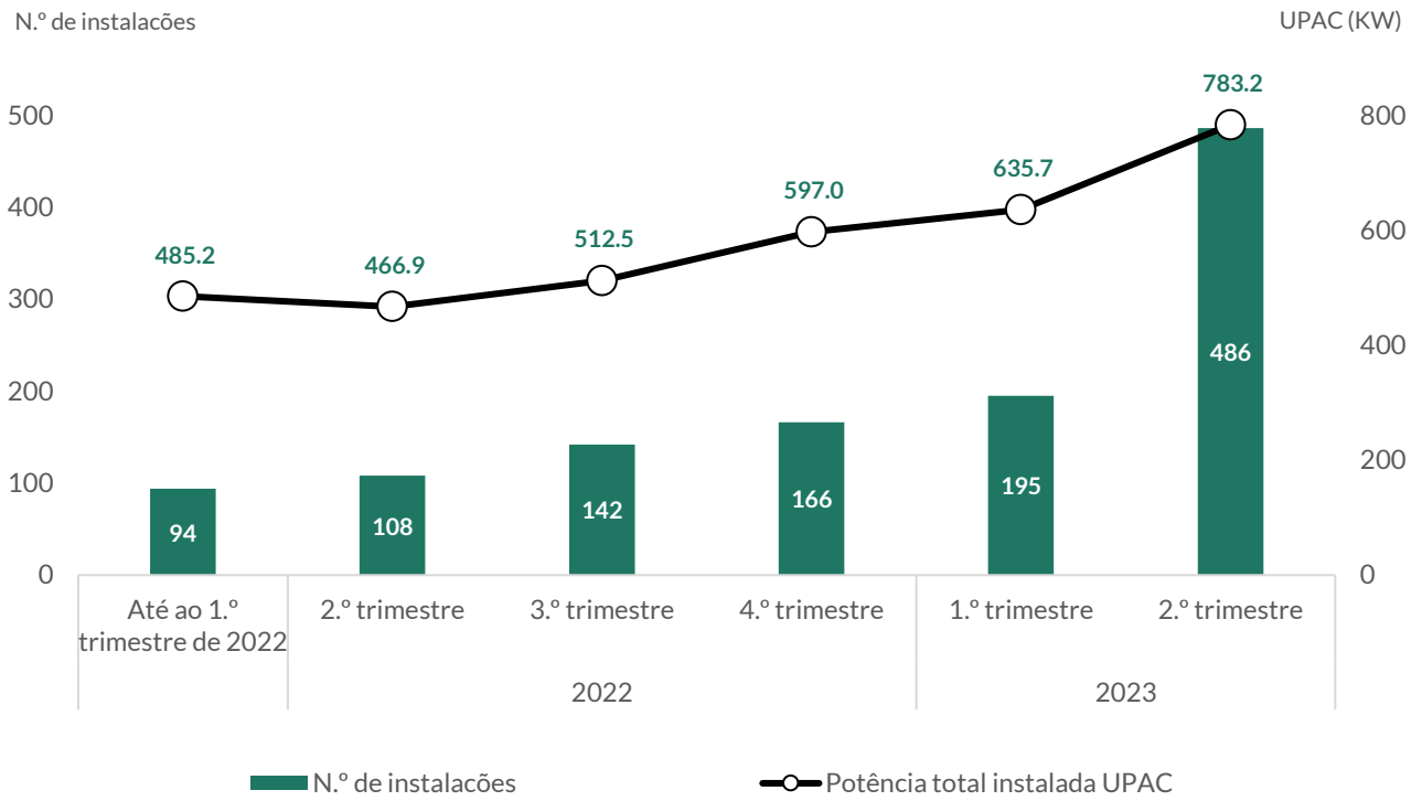
Gráfico 38 | Número de instalações e potência instalada de UPAC (acumulado), em Macedo de Cavaleiros, até ao 2º trimestre de 2023
